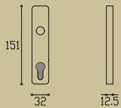
AM113PLY hef/schuifdeurbeslag sliding door fittings Hebeschiebetürgriffe
