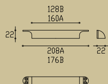
PA752RA PA752RB raamgreep window handle Fenstergriff
